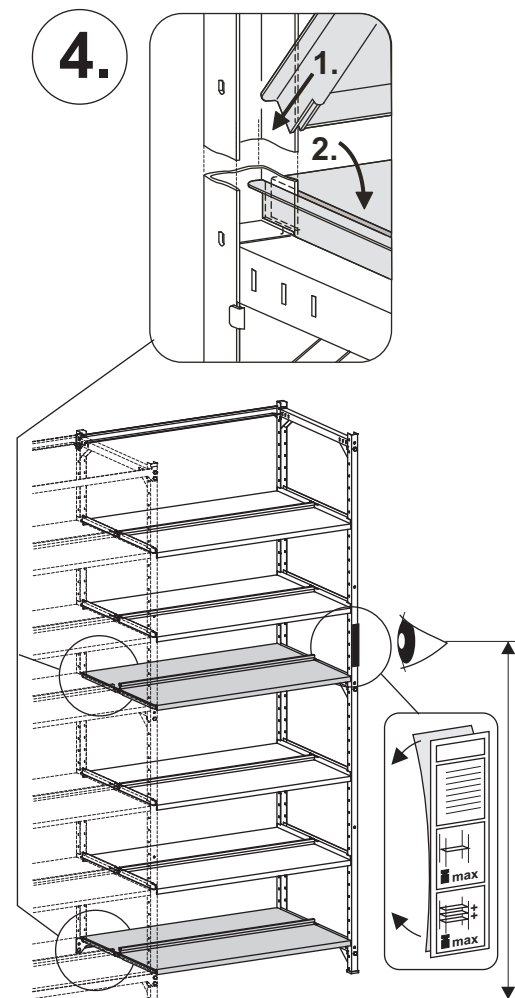
Megaflex Regi Verbinder Anbau 2250-600
