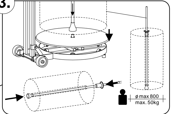
Senkrecht - Schneidständer
