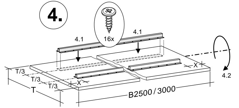
Arbeitstisch- Universal
